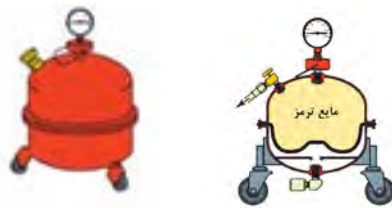
شکل ۱۶-۶- پر کردن و هواگیری سیستم هیدرولیک ترمز به وسیله دستگاه تزریق تحت فشار
