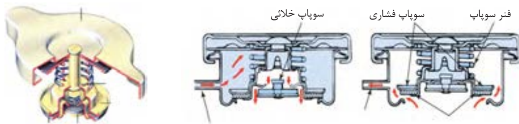
شکل ۷-۲۵- عملکرد در رادیاتور
