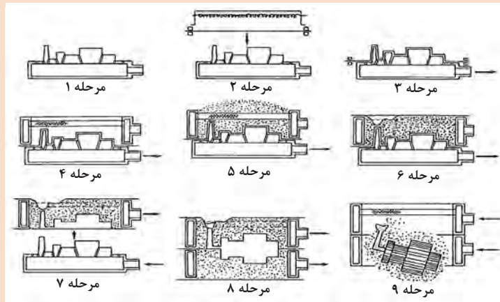
مراحل مختلف فرایند ریخته‌گری تحت خلأ
