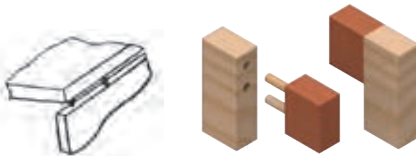
اتصال گوشه‌ای با دوپل مخفی
