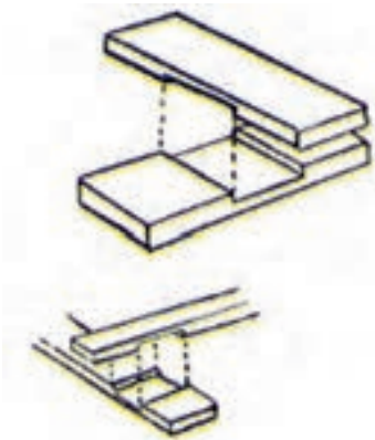
اتصال نیم صلیبی
