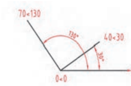
شکل ۶ - مختصات نقاط در سامانه مختصات قطبی
