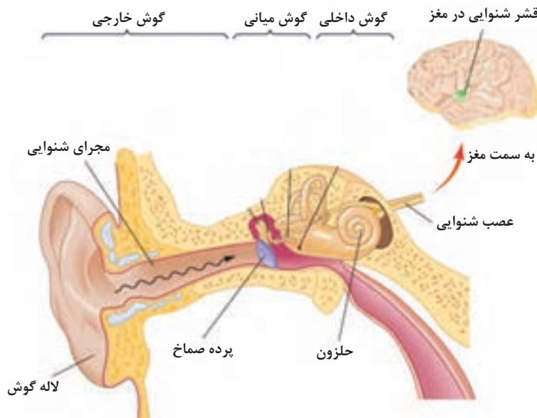
شکل ۲۱- ساختار گوش
