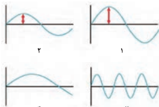
شکل ۲۲- امواج صوتی
